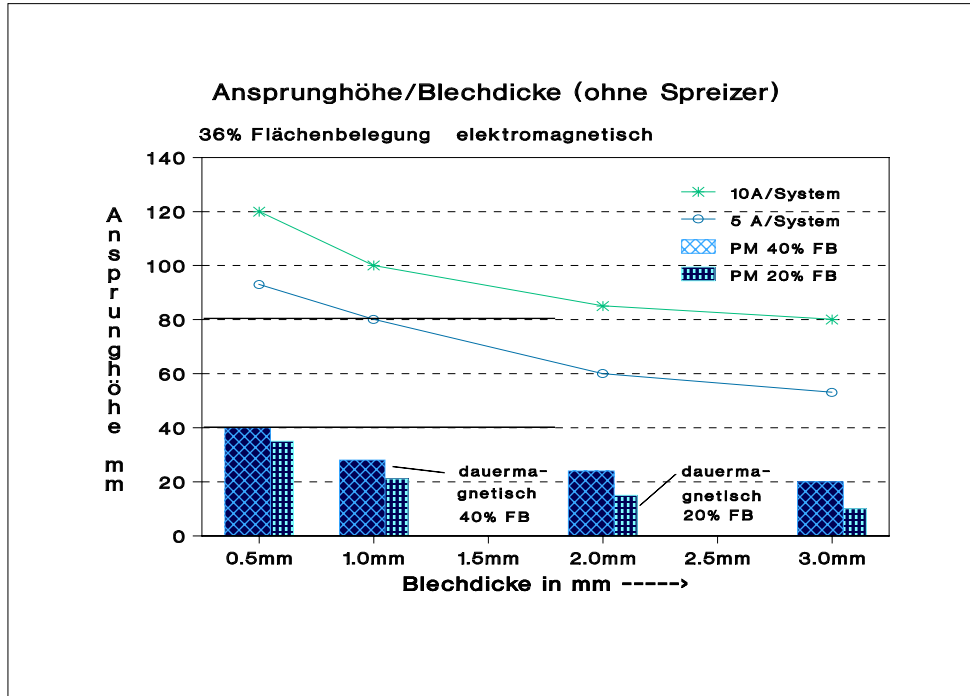
Bild 4: Ansrungshöhen des elektromagnetischen Systemteils im Vergleich zum permanentmagnetischen
