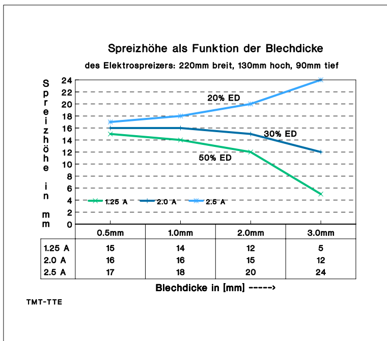
Bild 5: Die Spreizhöhe als Funktion der Blechdicke und des Spulenstromes
